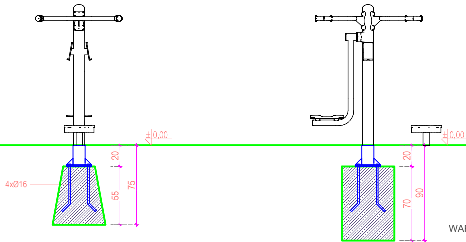
WARIANT 1 - FUNDAMENT PREFABRYKOWANY
