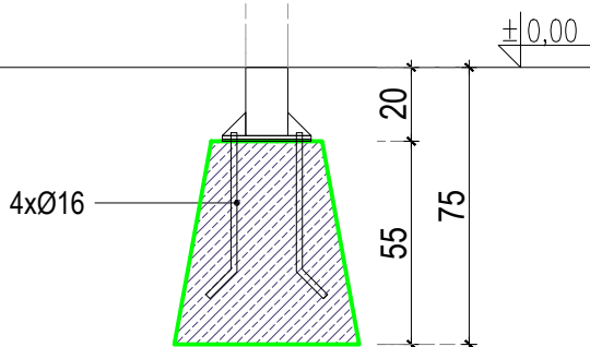
WARIANT 1 - FUNDAMENT PREFABRYKOWANY
