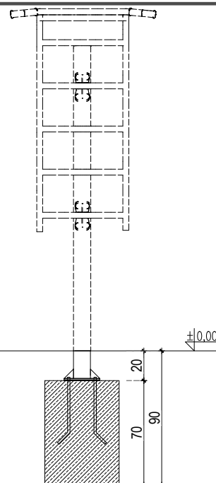
WARIANT 2 - FUNDAMENT WYLEWANY
